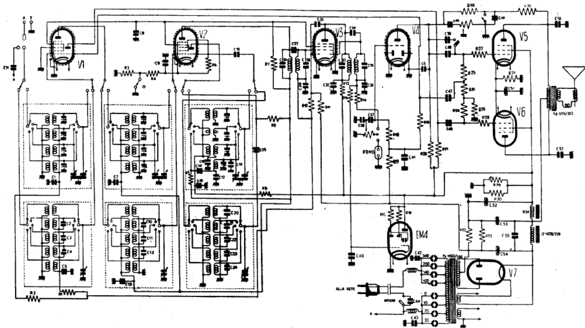
PHONOLA RADIO - Mod. 723 - Quattro gamme e cinque bande e spesse in onde corte come il mod. 722. Eccitazione altoparlante 120 V, massimo negativo - 2 V. MF a 470 kc. Consumo 105 W; potenza d'uscita 8 W.
